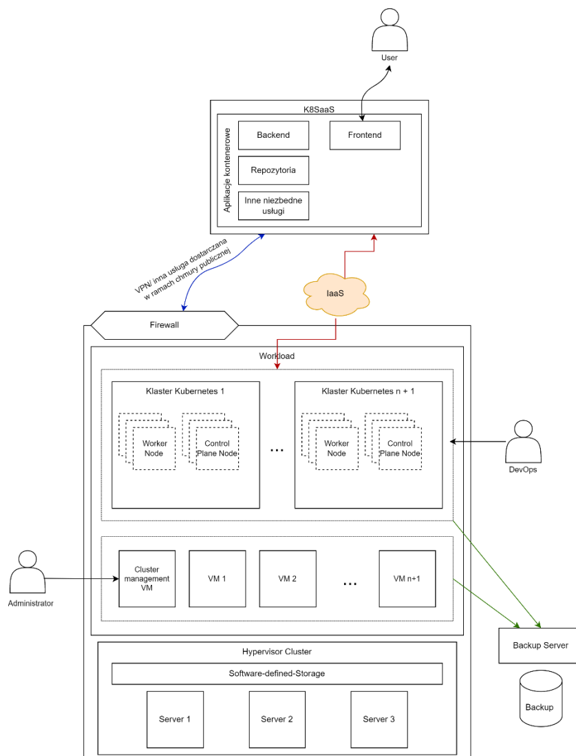
Rysunek 5 Schemat ogólny platformy do konteneryzacji.
