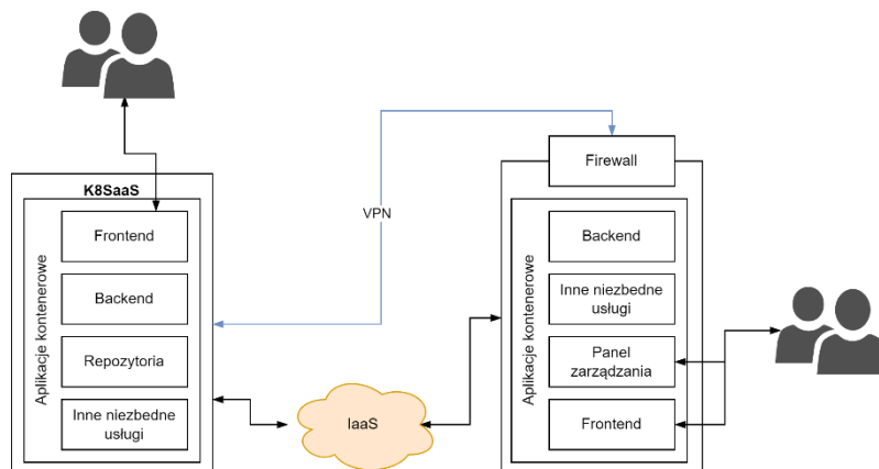
Rysunek 2 Ogólny schemat połączenia WAN
