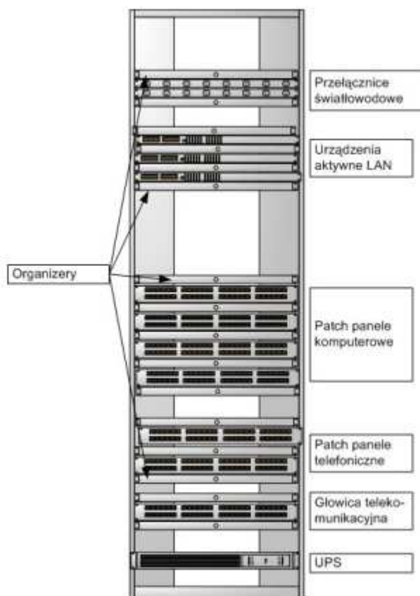
Rys.1: Sposób rozmieszczenia elementów aktywnych i pasywnych w szafie.
